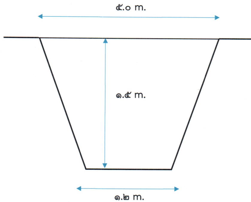
รูปที่ ๖ ขนาดรางระบายน้ำจุดที่ ๕
