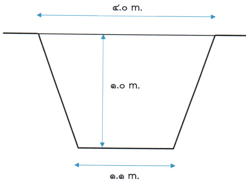
รูปที่ ๓ ขนาดรางระบายน้ำจุดที่ ๒
