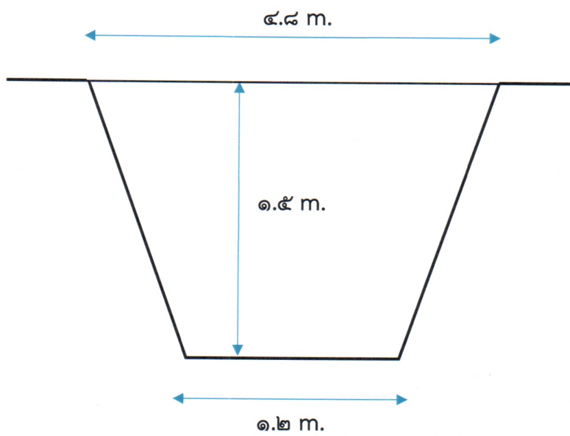
รูปที่ ๔ ขนาดรางระบายน้ำจุดที่ ๓
