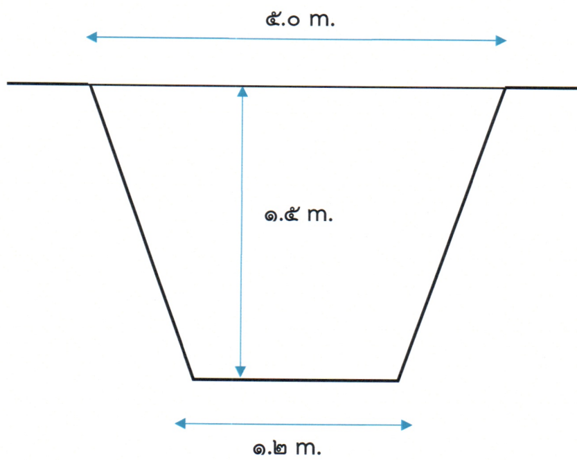
รูปที่ ๕ ขนาดรางระบายน้ำจุดที่ ๔
